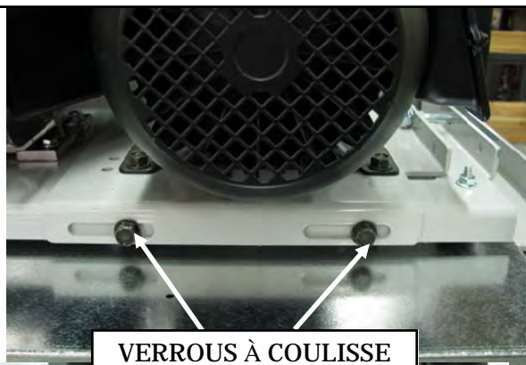
VERROU D'AJUSTEMENT DE LA COURROIE
