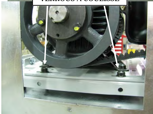
VERROUS À COULISSE
